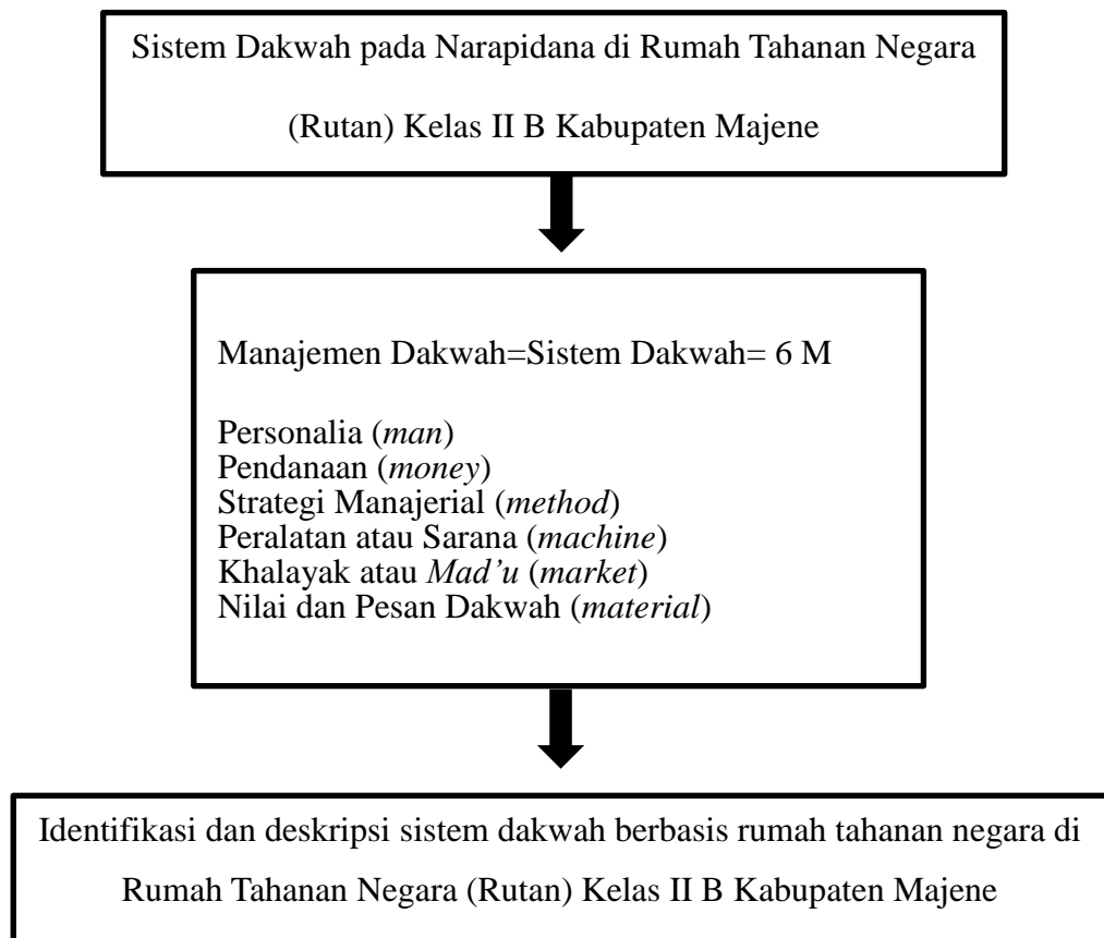
Gambar 3.1. Kerangka Konseptual
