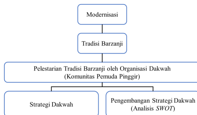
Gambar 2.1 Kerangka Konsep
