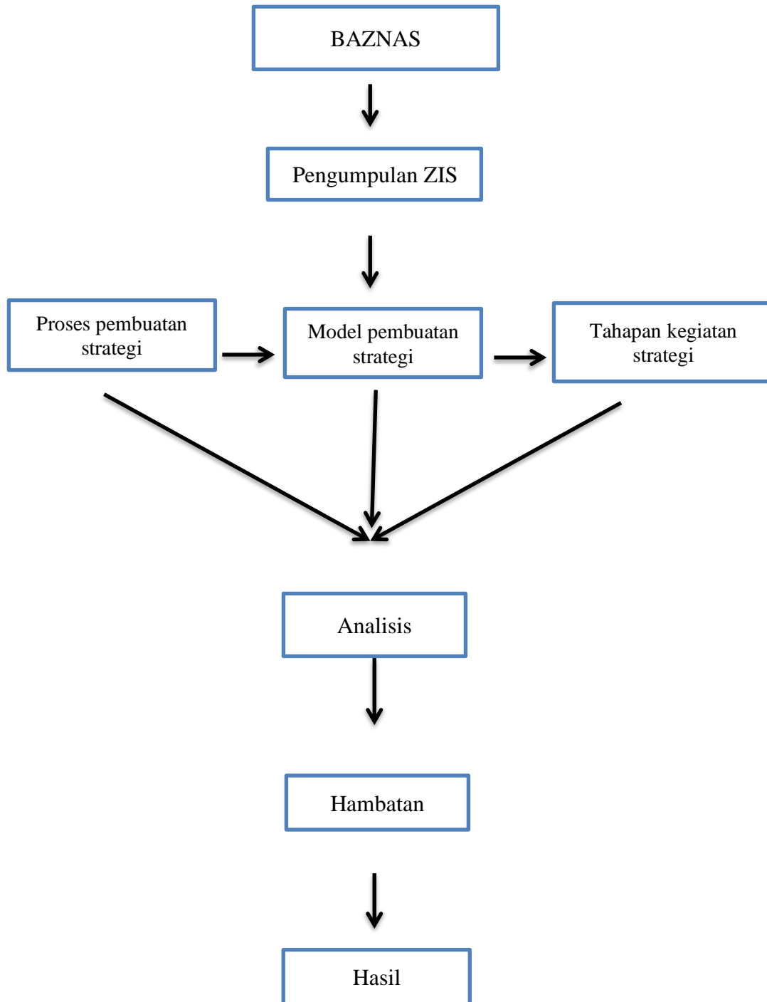
Gambar. 1.1 Kerangka Penelitian
