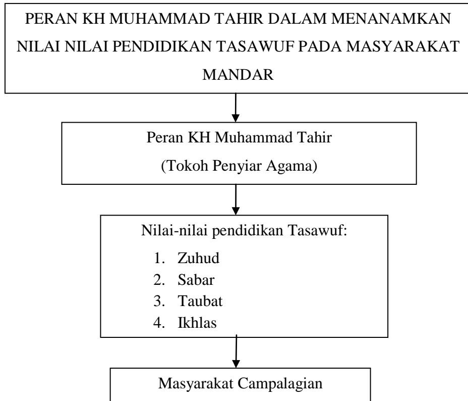
Gambar 1.1 Kerangka Konseptual
