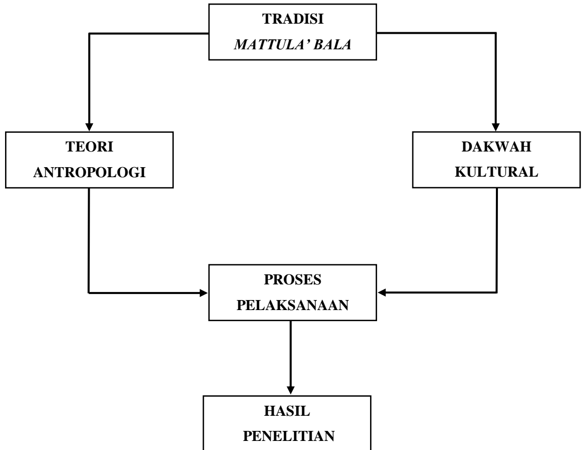
Gambar. 1 Kerangka Konseptual
